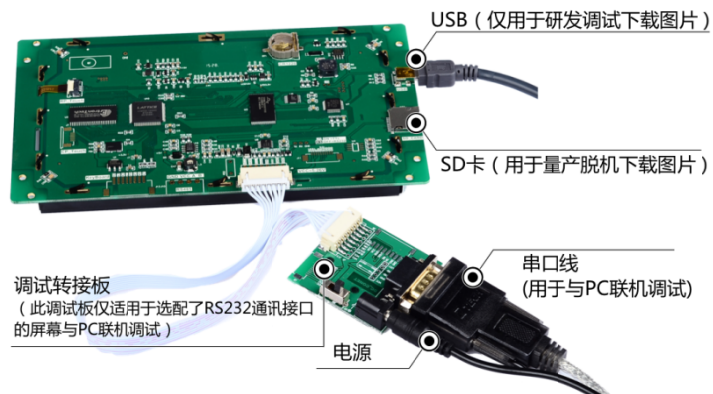
图 1-5 调试工具图
