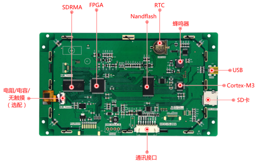
图 1-4 硬件配置图
